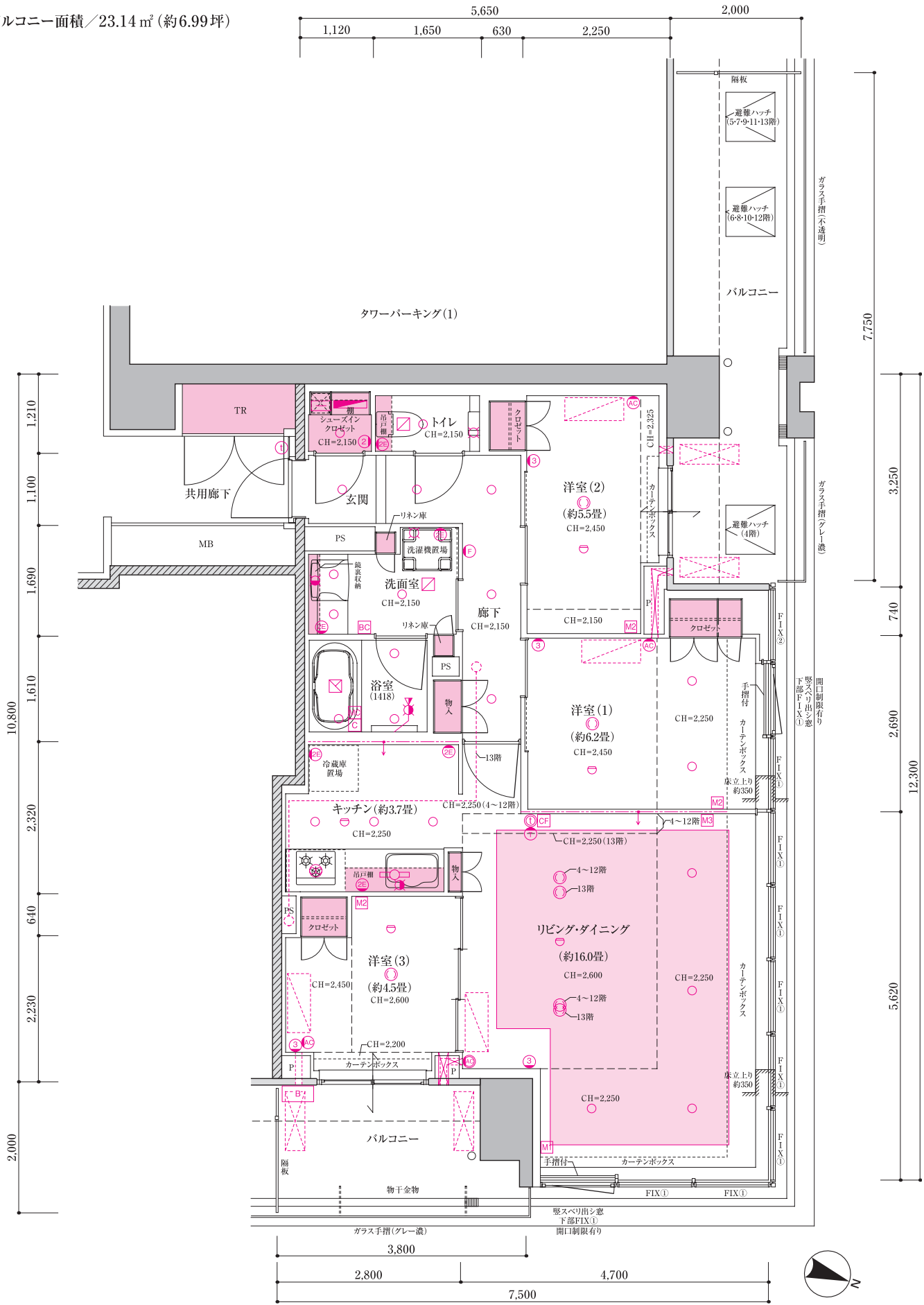
■ 13 階部分図 Scale: 約 1/80
