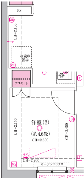
28 階部分図 Scale: 約 1/80
