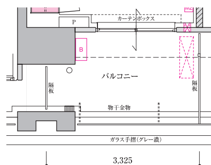
■ 4 階部分図 Scale: 約 1/80
