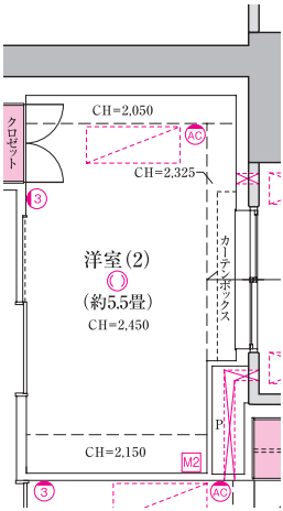
■ 13 階部分図 Scale: 約 1/80
