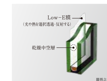
Low-E 複層ガラス ■概念図
