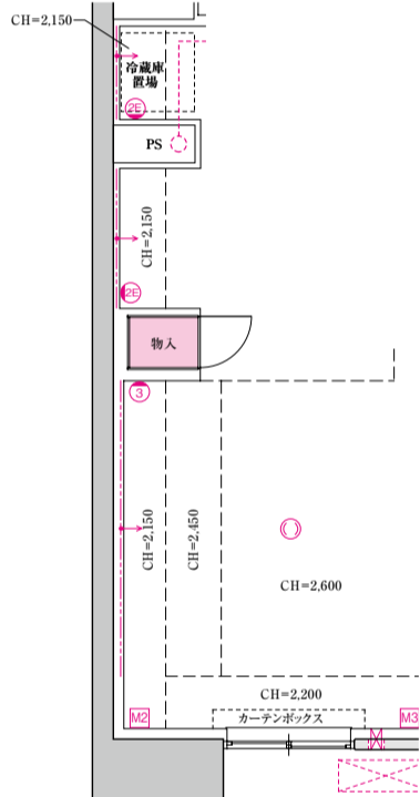
■ 28階部分図 Scale: 約1/80
