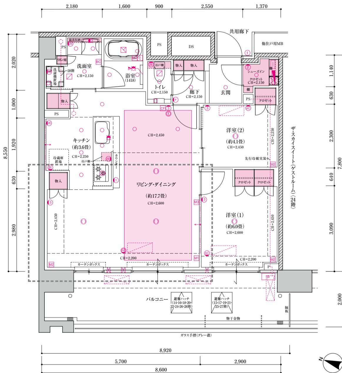
■ 28階部分図 Scale:約1/80
